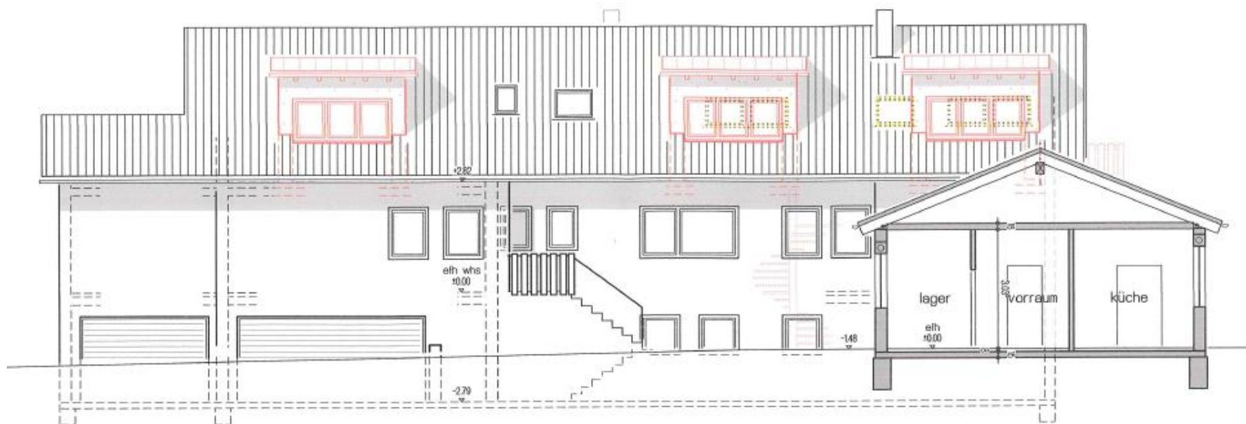
schnitt b-b mit ansicht nordost
